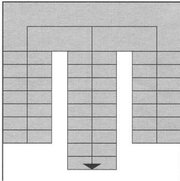
Dreiläufige gegenläufige Treppe mit Zwischenpodest
