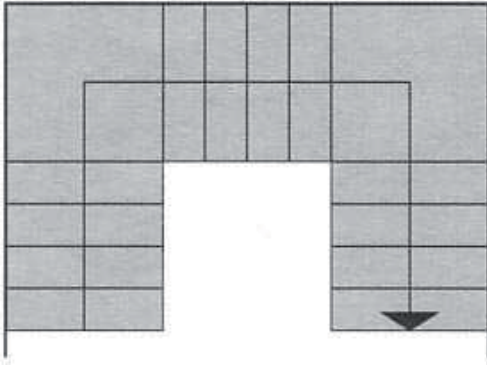
Dreiläufige zweimal abgewinkelte Treppe mit Zwischenpodesten
