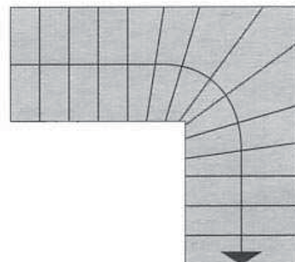
Einläufige gewinkelte viertelgewendelte Treppe
