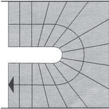
Einläufige, halbgewendelte Treppe
