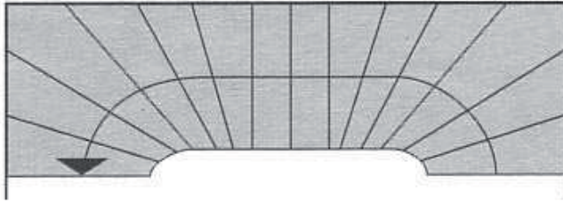
Einläufige, zweimal viertelgewendelte Treppe
